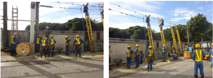
ハンガ取替 区分がいし取替 昇降練習
